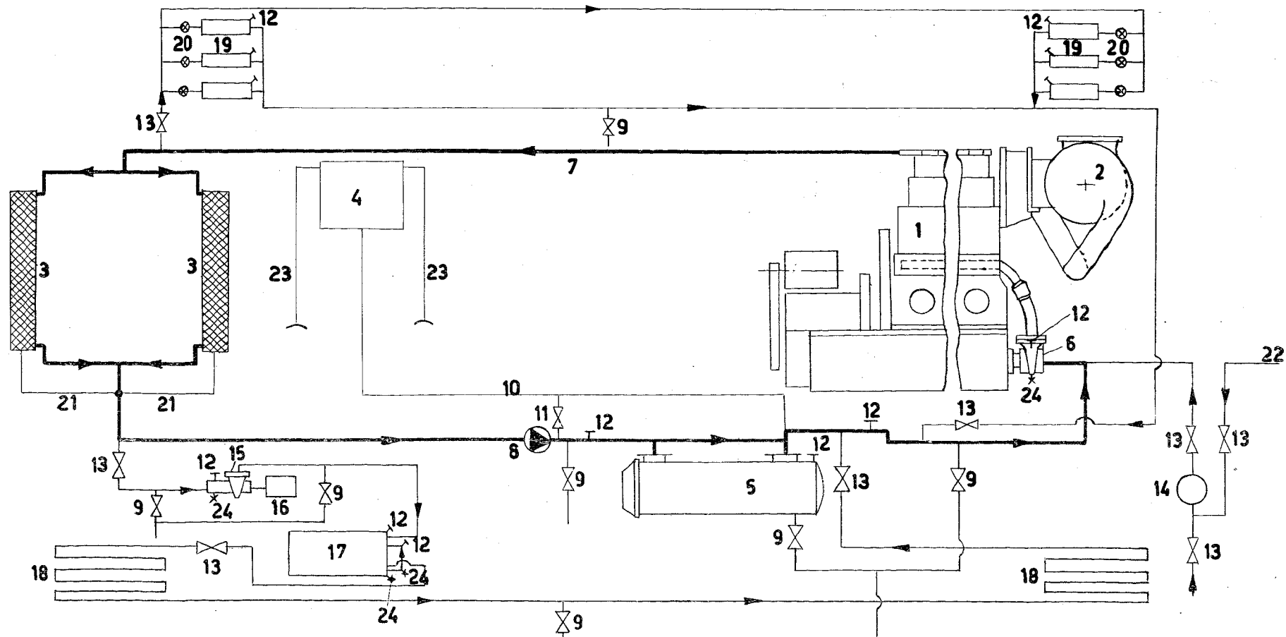
SCHEMA VAN DE WATEROMLOOP
