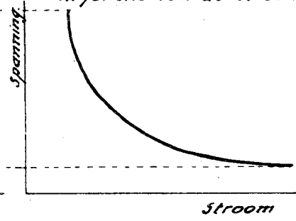
Fig. III /4. ELECTRISCHE OVERBRENGING MET CONSTANT VERMOGEN.
