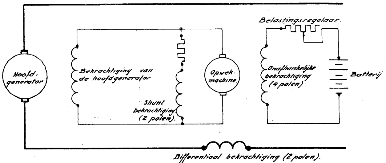
Fig. III /6. PRINCIEP VAN DE REGELING VAN HET VERMOGEN.
