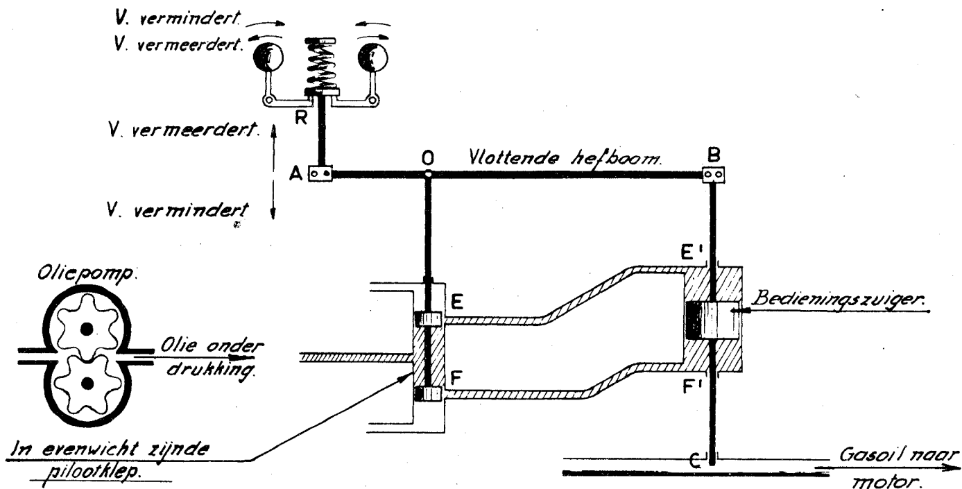
Fig. II / 18. NORMALE STAND VOOR EEN BEPAALDE BELASTING.
