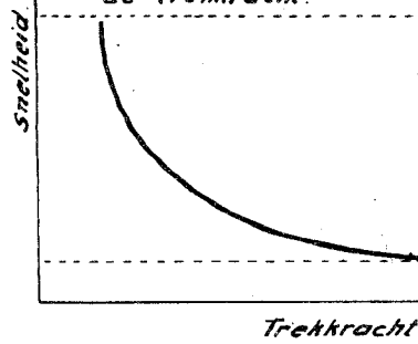
Fig. III /4. ELECTRISCHE OVERBRENGING MET CONSTANT VERMOGEN.
