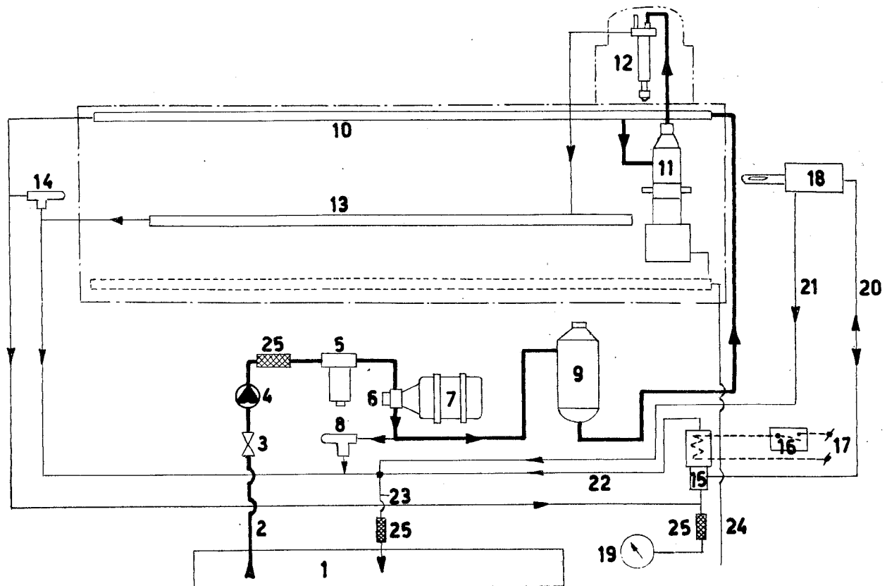
SCHEMA VAN DE BRANDSTOFOMLOOP
